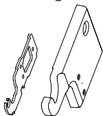
Oberes linkes Schar- nier (Türanschlag kann umgekehrt werden)
